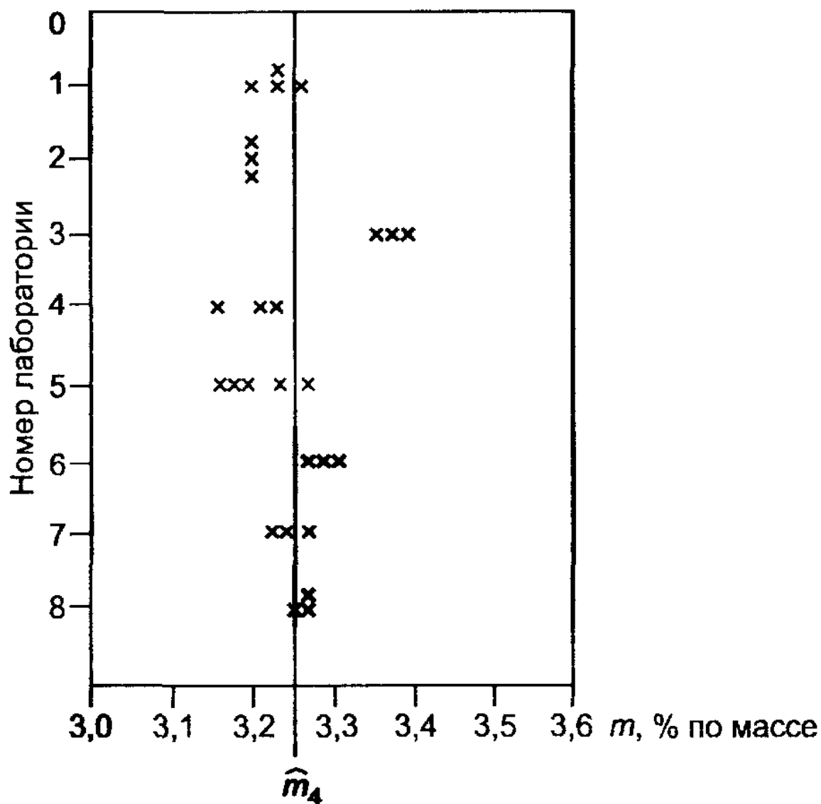
Рисунок В.4 — Содержание серы в угле, уровень (образец) 4
