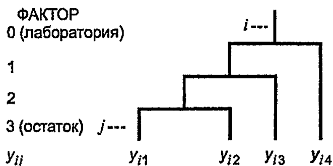
Рисунок 2 — Схема четырехфакторного ступенчато вложенного эксперимента
