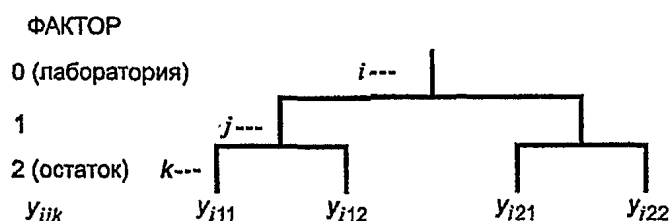
а) трехфакторный полностью вложенный эксперимент
