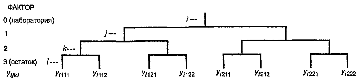
б) четырехфакторный полностью вложенный эксперимент
