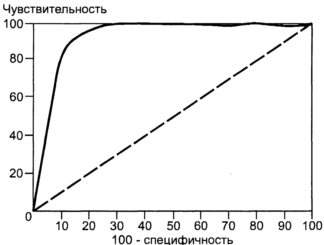
Рисунок 3 — ROC-кривая
