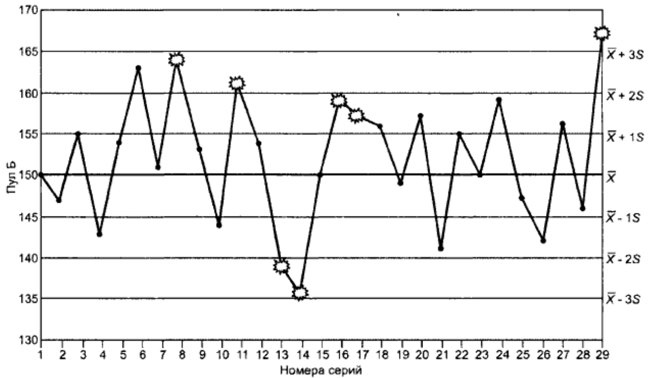
Рисунок 3 — Примеры нарушения контрольных правил в случае двух контрольных материалов
