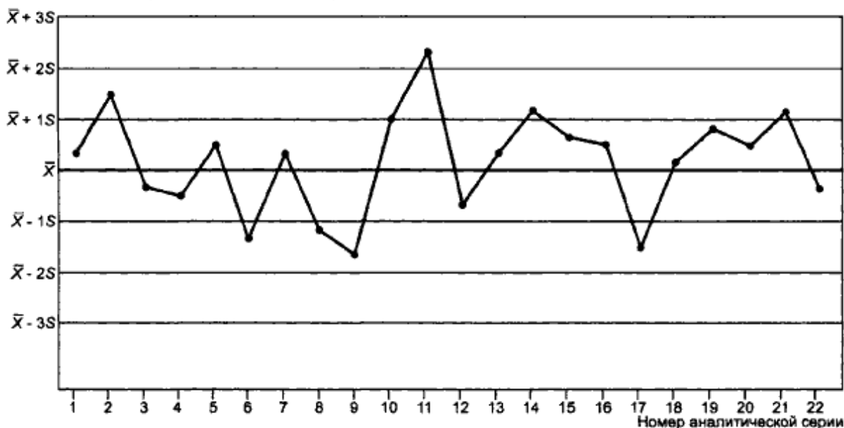
Рисунок 1 — Пример контрольной карты
